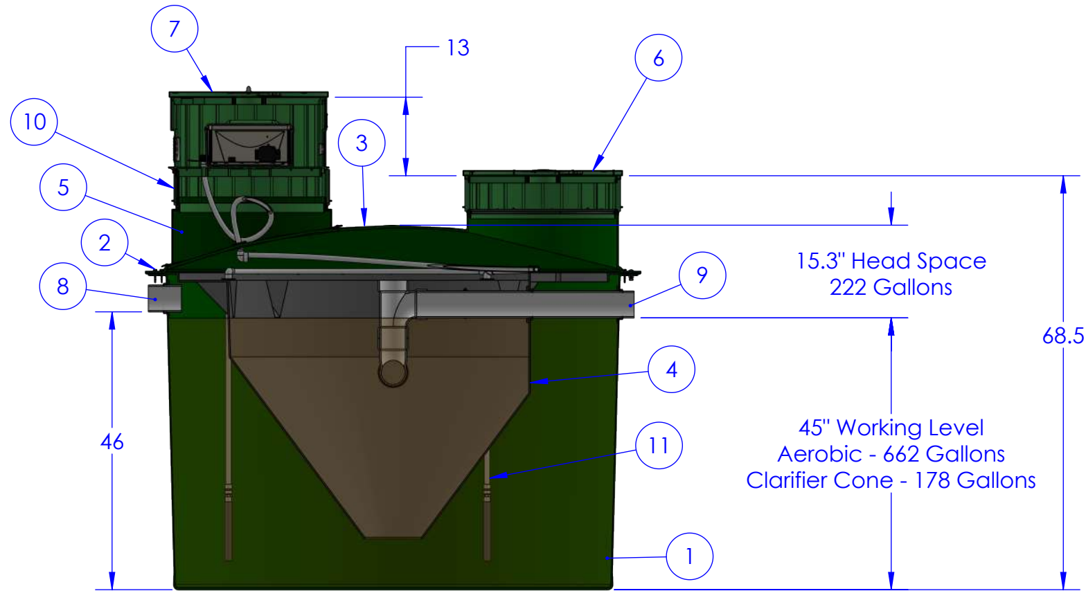
SECTION A-A SCALE 1 : 22
