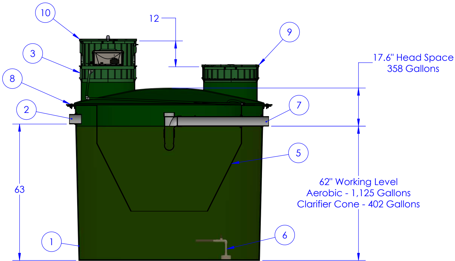
SECTION A-A
